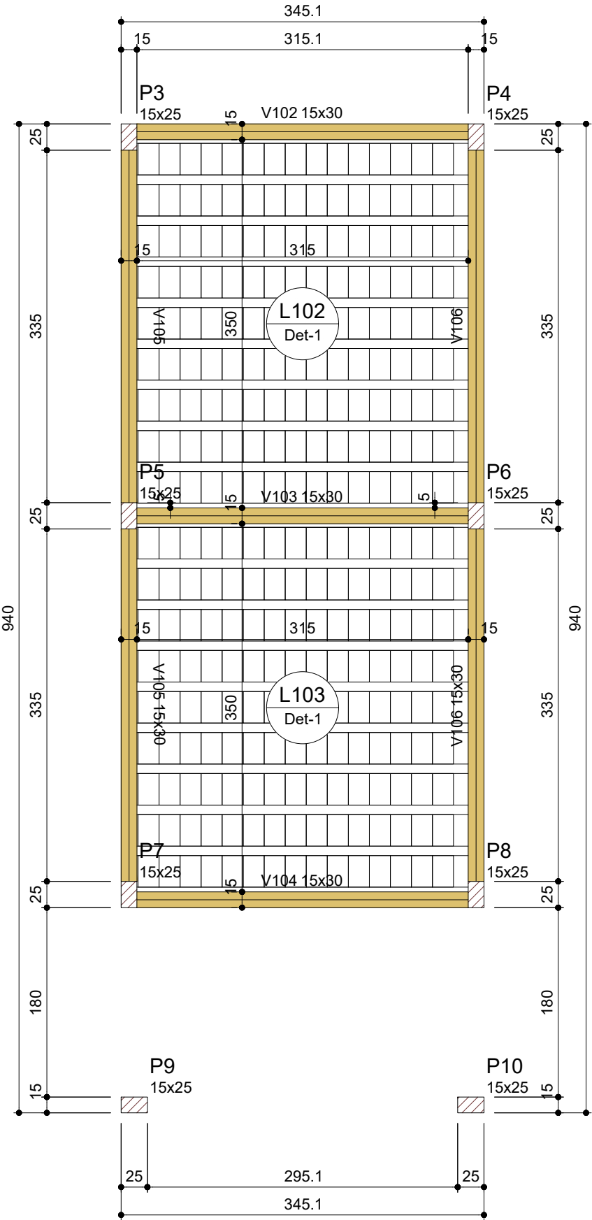
Forma do pavimento Térreo (Nível 290) escala 1:50
