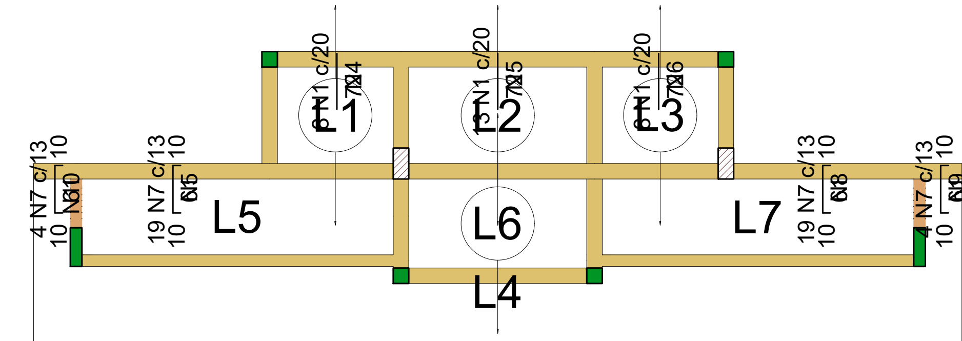
Armação negativa das lajes do pavimento Laje (Eixo Y) escala 1:50
