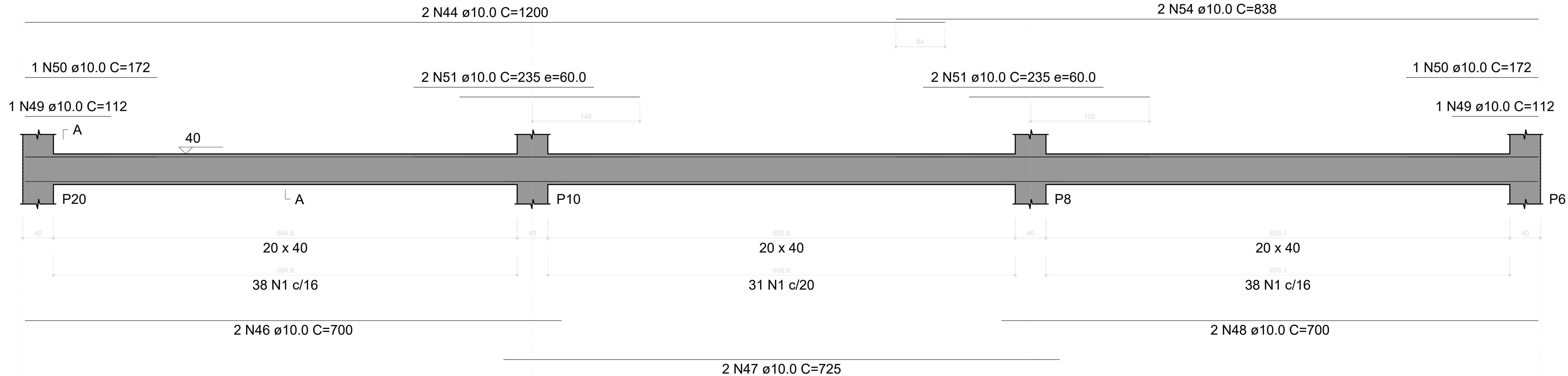
V14 ESC 1:30
