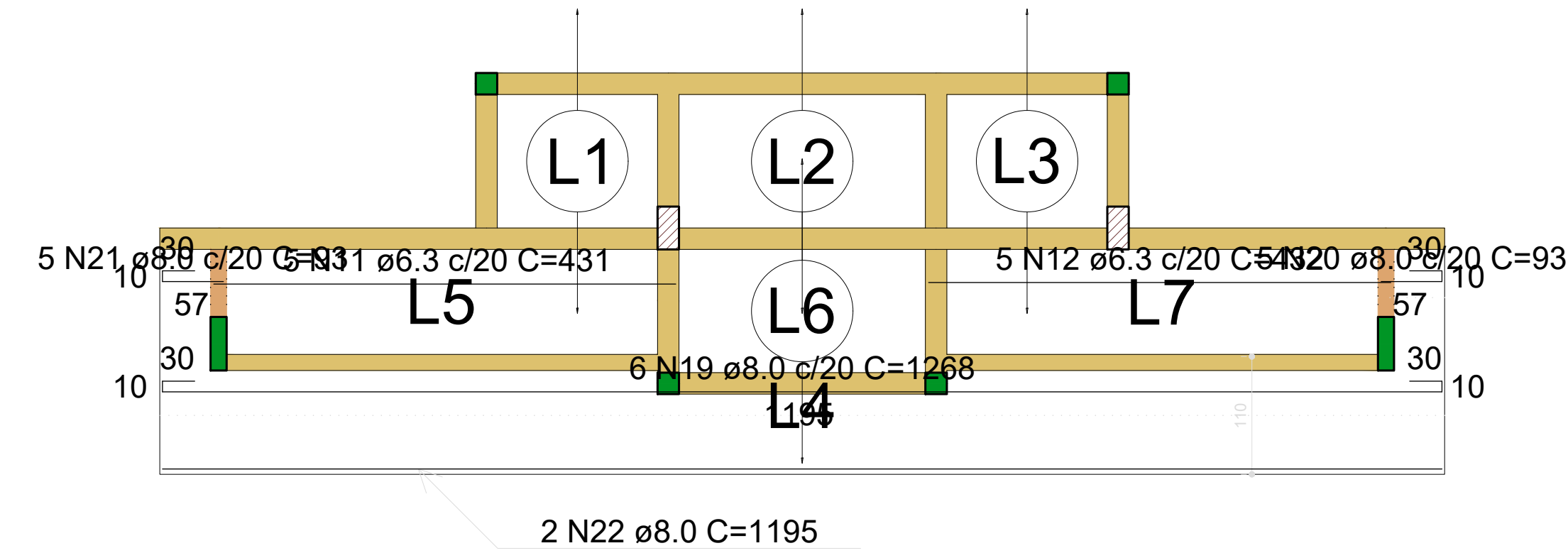
Armação positiva das lajes do pavimento Laje (Eixo X) escala 1:50
