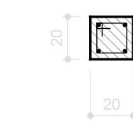
SEÇÃO A-A ESC 1:25
