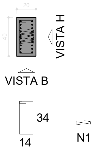
SEÇÃO ESC 1:20
