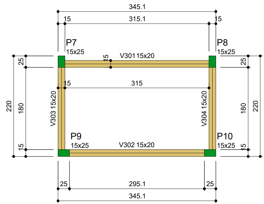
Forma do pavimento Platibanda (Nível 455) escala 1:50
