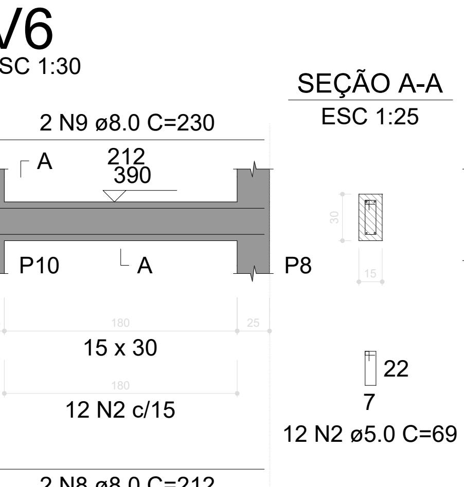
SEÇÃO A-A ESC 1:25
