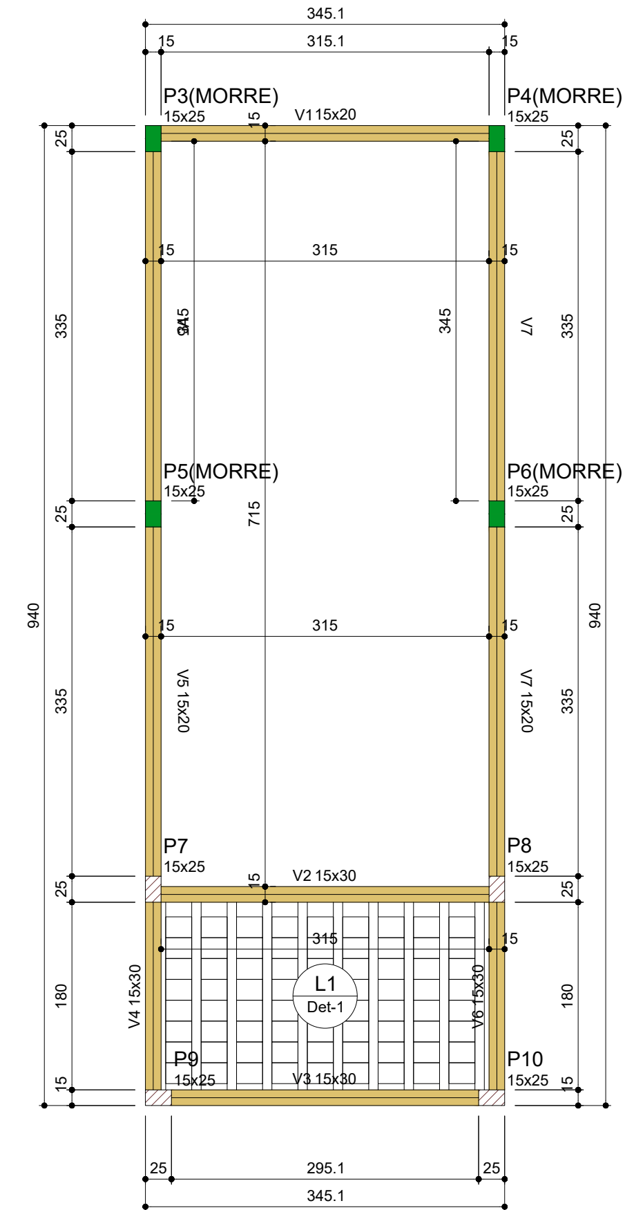
Forma do pavimento Fundo de Caixa d'água (Nível 390) escala 1:50
