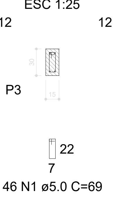
SEÇÃO A-A ESC 1:25
