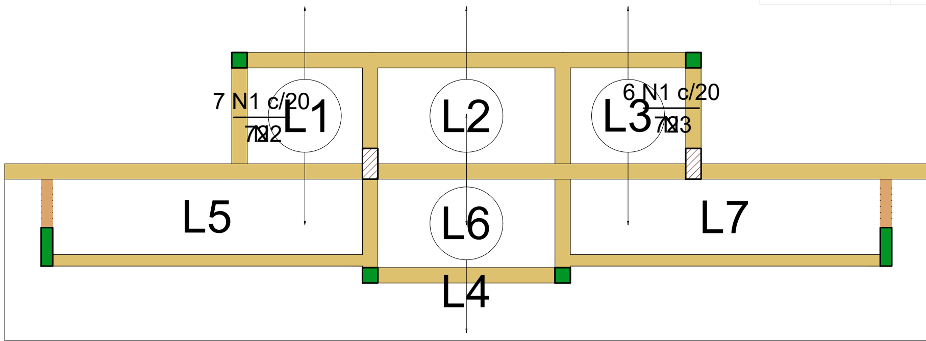
Armação negativa das lajes do pavimento Laje (Eixo X) escala 1:50
