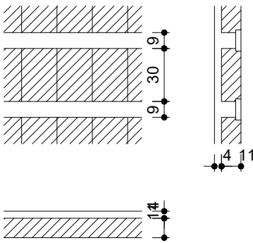
Detalhe 1 (esc. 1:30)
